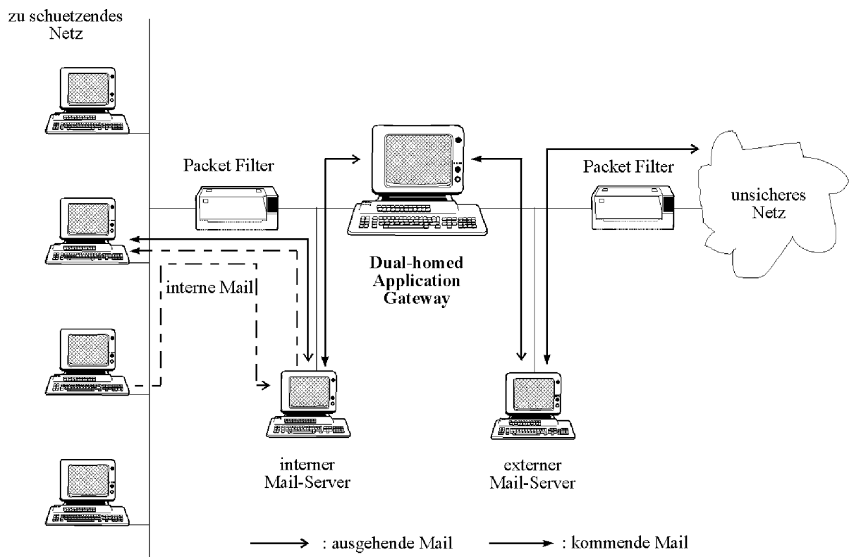
Abb.5: Anordnung der Mail-Server
