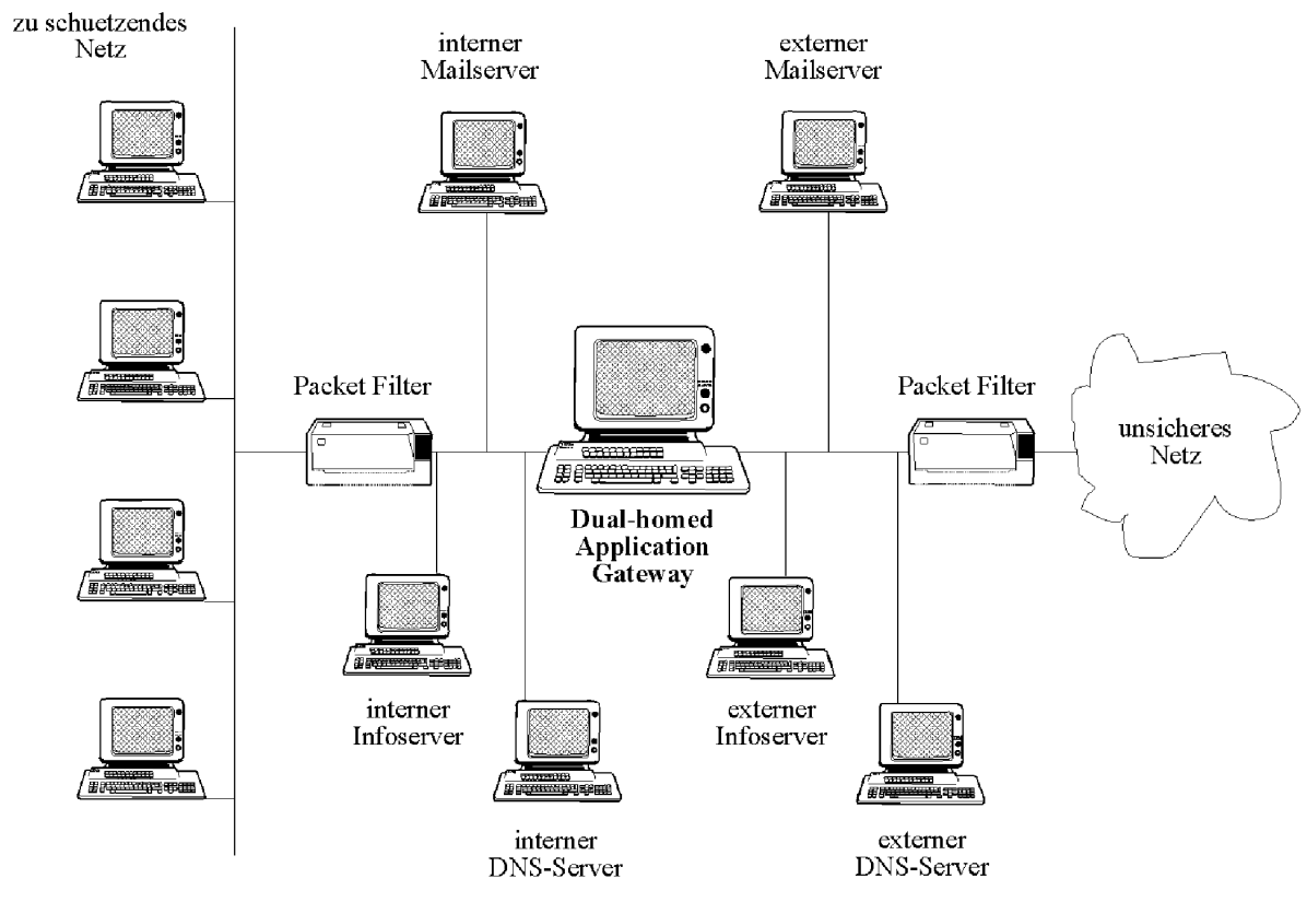
Abb. 4: Screened Subnet mit Dual-homed Gateway
